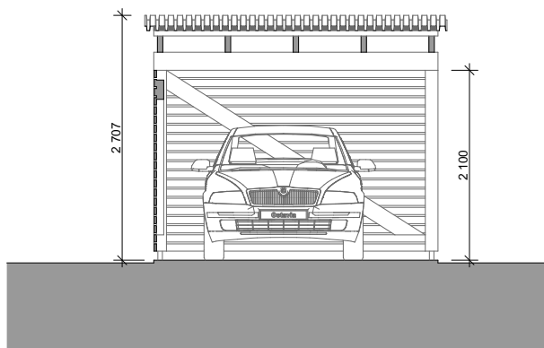
PŘÍČNÝ ŘEZ 1:75
