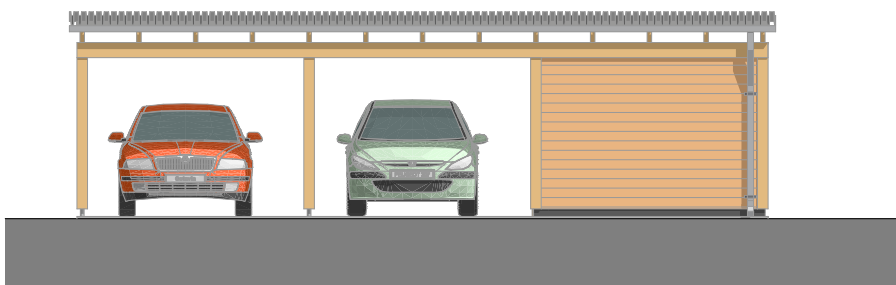
BOČNÍ POHLEDY 1:100
