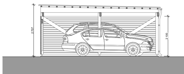
SVISLÉ ŘEZY 1:100
