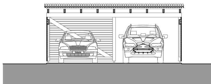
SVISLÉ ŘEZY 1:100
