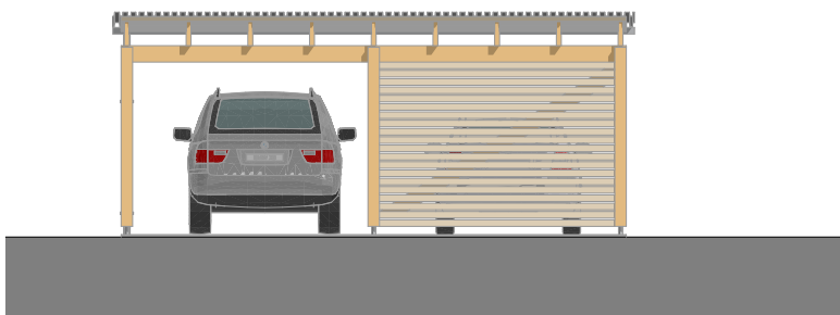
BOČNÍ POHLEDY 1:100
